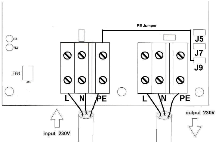
Abb. 2: Eingangserdung
